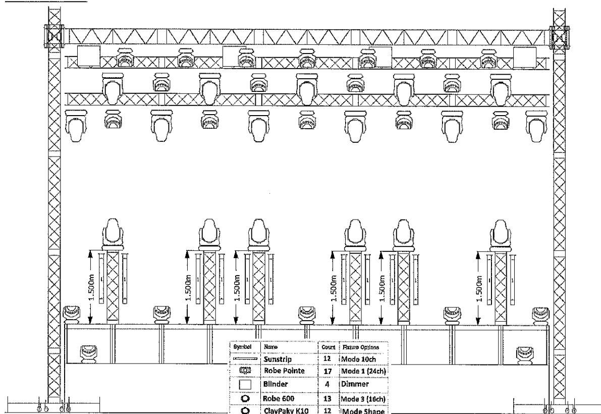
RZUT FRONT
